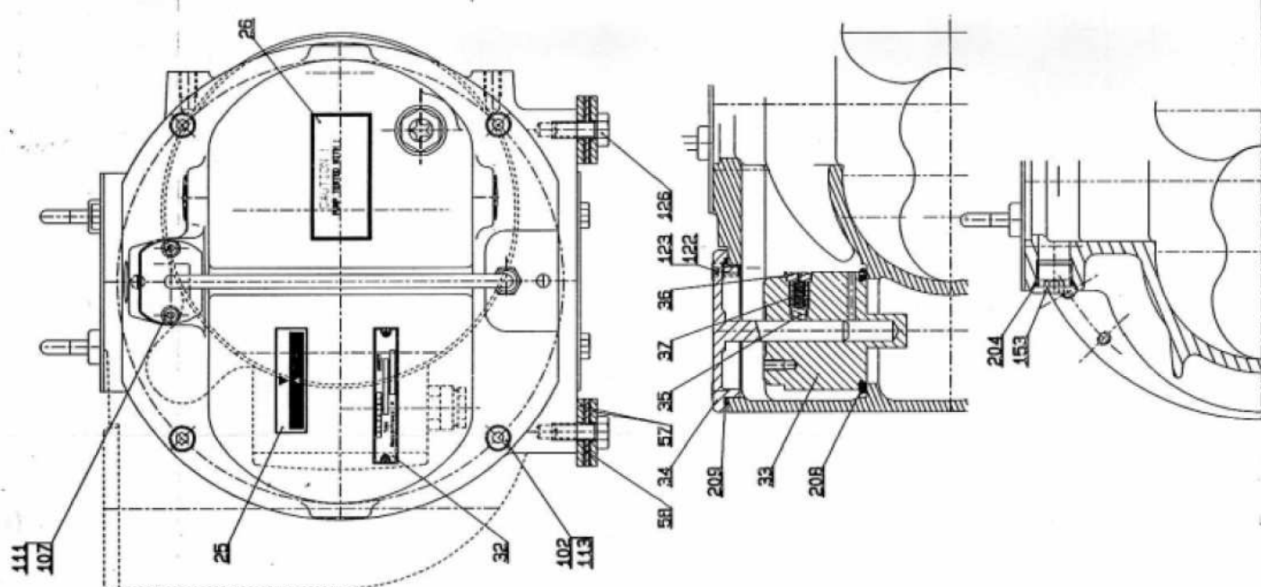
ROOTS RSV 301/301 B/601/601B PLAN D'ENSEMBLE/GENERAL DRAWING ÜBERSICHTPLAN
